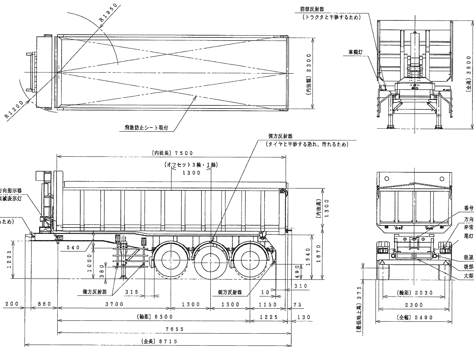
コダイラ KDA315C ダンプセミトレーラ外観図
