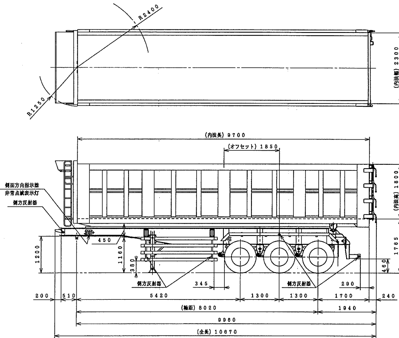
コダイラ KFL32改 ダンプセミトレーラ外觀四面図 (KFL32-1224)
