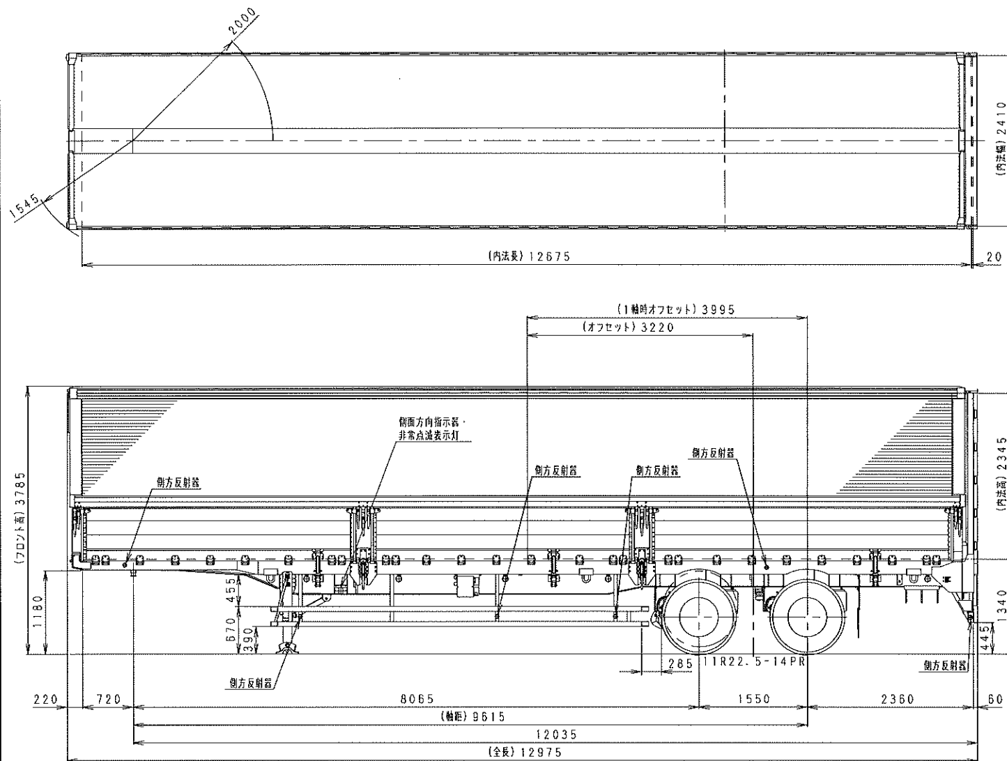
東 邦TF28H7B2改型 バンセミトレーラ外觀四面図
