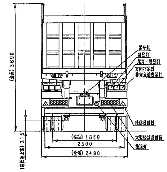
東邦TF36H2C3型 セミトレーラ外観四面図
