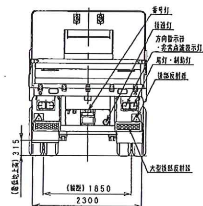
東急TF36H2C3型 セミトレーラ外觀四面図 Y-48397
