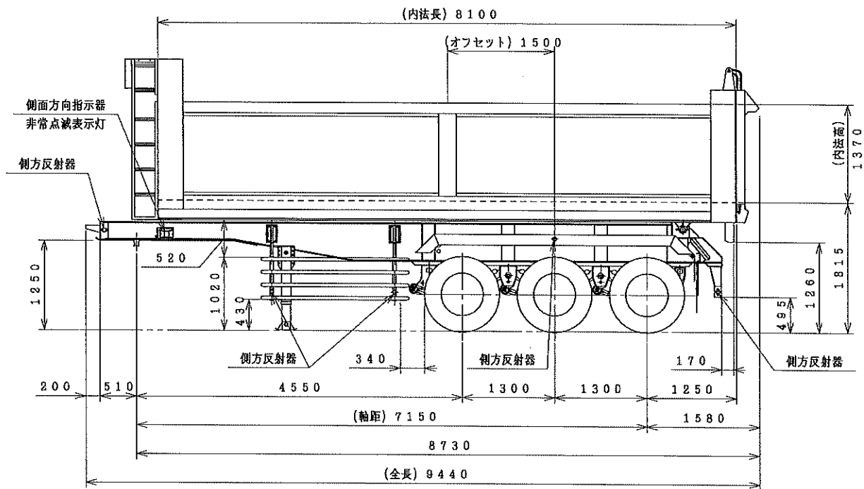
コダイラ KFL32改 ダンプセミトレーラ外觀図 (KFL32-2096、KFL32-2097)
